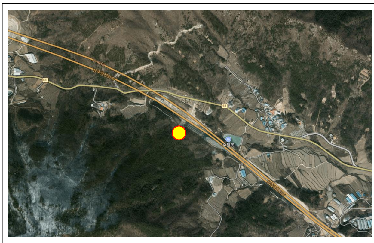
【그림 18.13】 영천절토18 검토대상 비탈면구간
