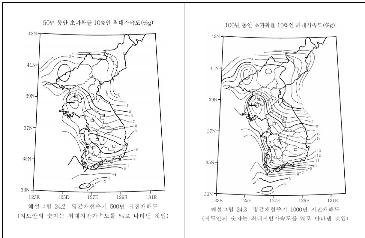
【그림 18.12】 평균재현주기 500년 및 1000년 지진재해도
